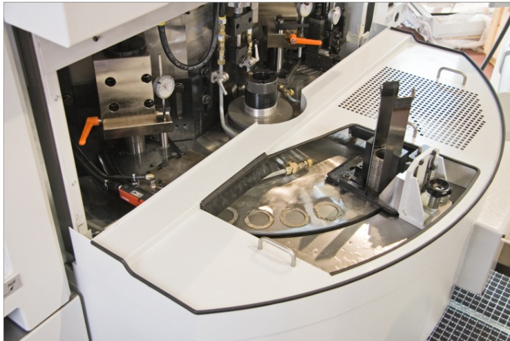
Bild 1: Supfina Planet V mit Magazin.
