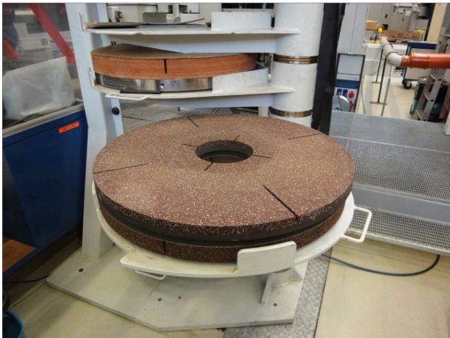
Bild 6: Optimal ausgelegte Schleifscheiben beeinflussen das Schleifergebnis maßgeblich.
