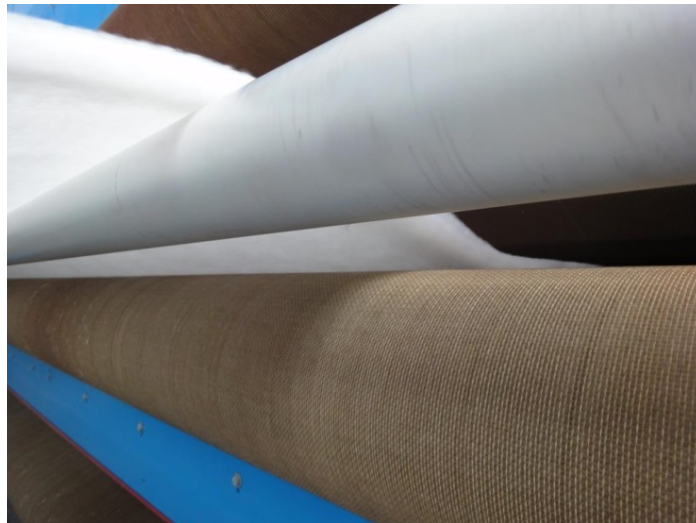
Bild 7-8: Maßgeschneidertes Trocknerband von GKD erfüllt die besonderen Anforderungen der dicken Dämmprodukte.
