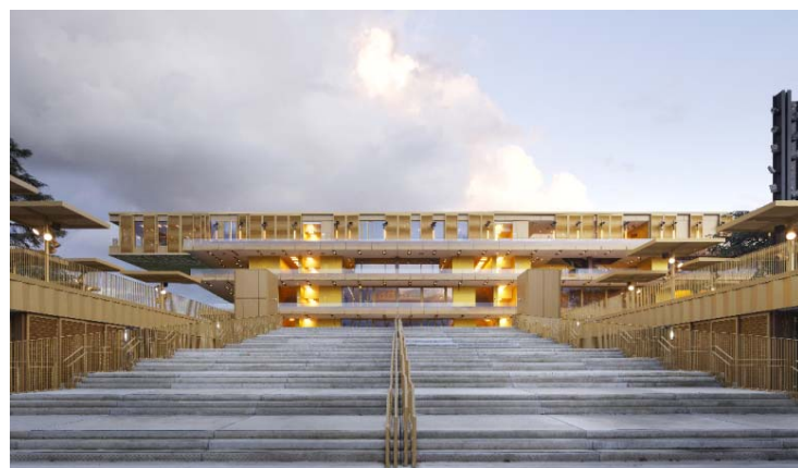
Photo 3 : Une maille inox dorée de type ESCALE 7x1,5 a été choisie pour les éléments de protection thermique de la tribune et des pavillons qui flanquent l'entrée principale de ParisLongchamp.
